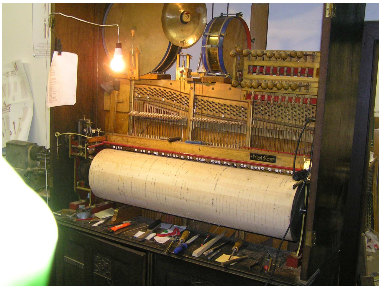
Ochestraion fy Klepetář, velký model po gen. opravě – výroba nového hracího válce, r. 2006.
